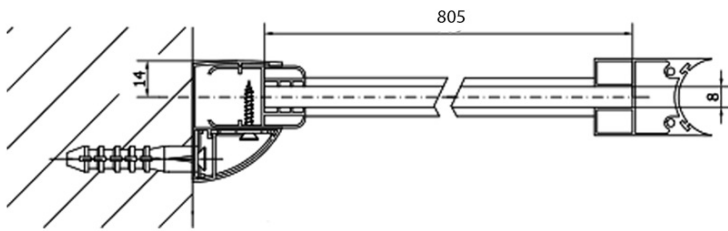
MS3A-90L
